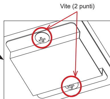
Protezione per scatola di comando (N. 8)
