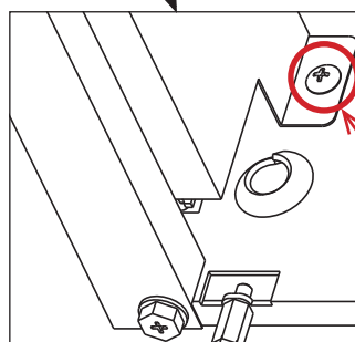
Vite (2 punti in alto e in basso)
