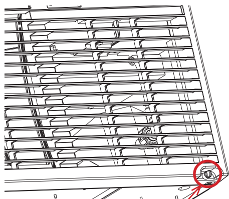
Vis à oreilles (2 points)
